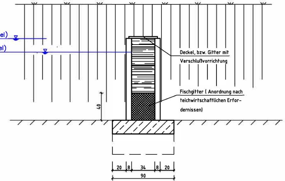
SCHNITT B-B
