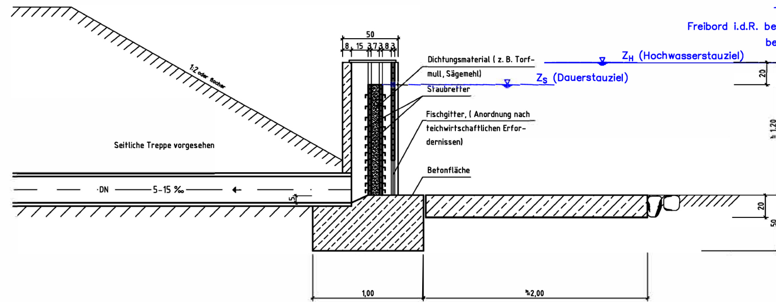
SCHNITT A-A
